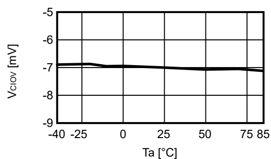
2. 12 V_{\text{CI OV}} - T_a
