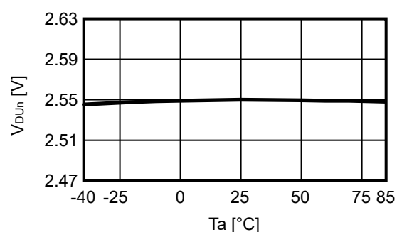
2.4 V_{DUN} - T_a
