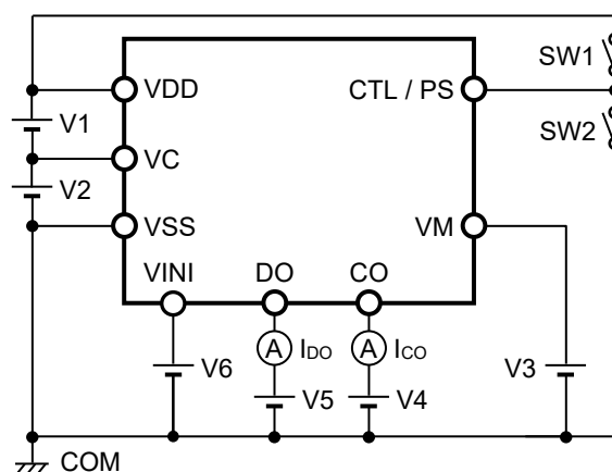
図8 測定回路4
