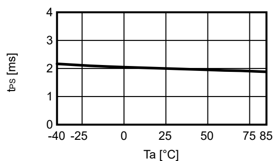
3. 14 t_{PS} - T_a (S-82A2Bシリーズ)
