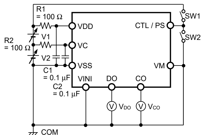
図5 測定回路1
