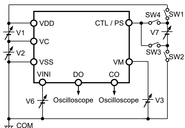
図9 測定回路5
