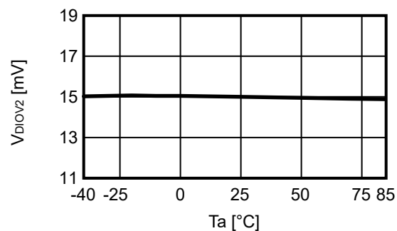
2.8 V_{DIOV2} - T_a
