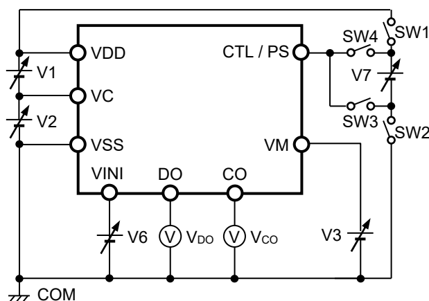
図6 測定回路2
