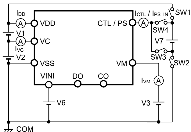
図7 測定回路3
